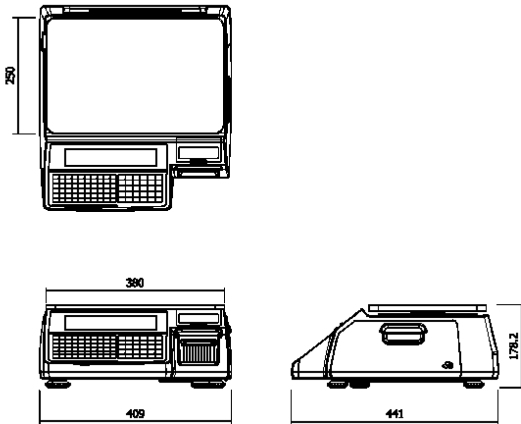
Рисунок 1.2 – Вид весов CL3000-B в геометрической проекции
