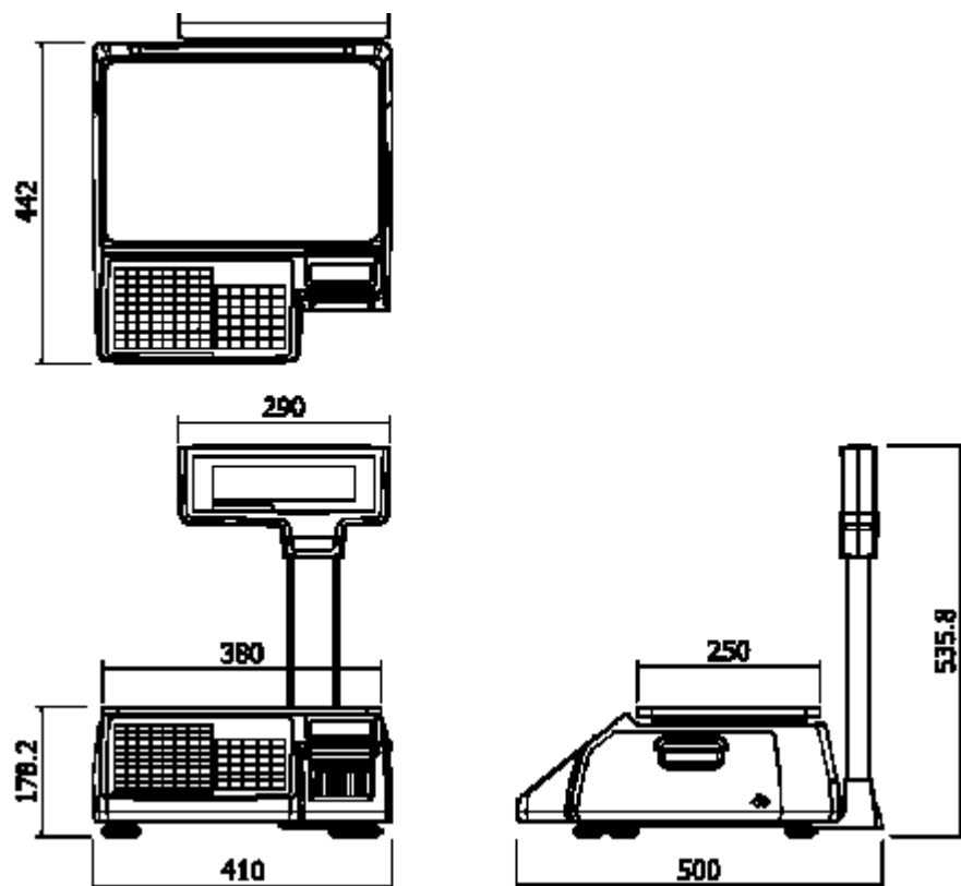
Рисунок 1.3 – Вид весов CL3000-P в геометрической проекции
