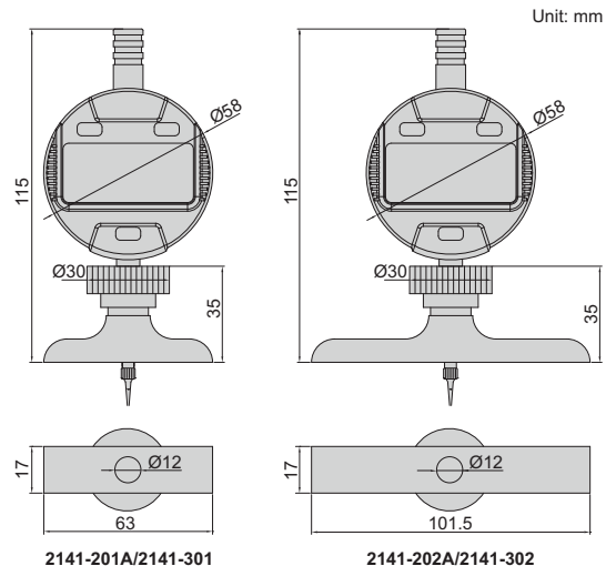
2141-201A/2141-301
