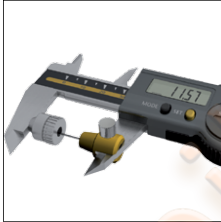
S-Cal с набором 910.2207 Измерение глубины в малых отверстиях
